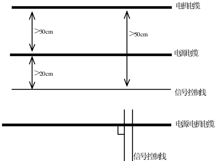
图 4-7 现场配线示意图
