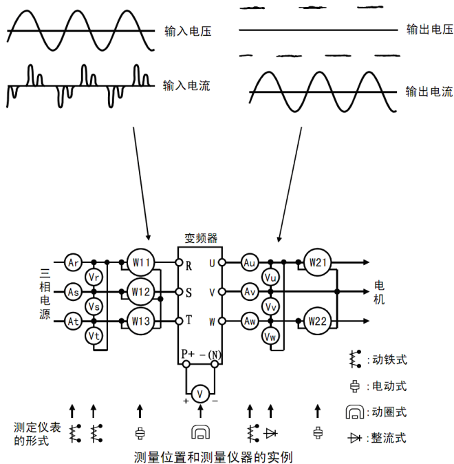
图 4-3 测量示意图
