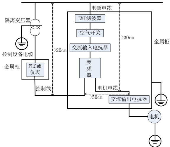
图 4-9 电气安装示意图
