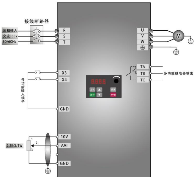
图 5-3 接线图 3
