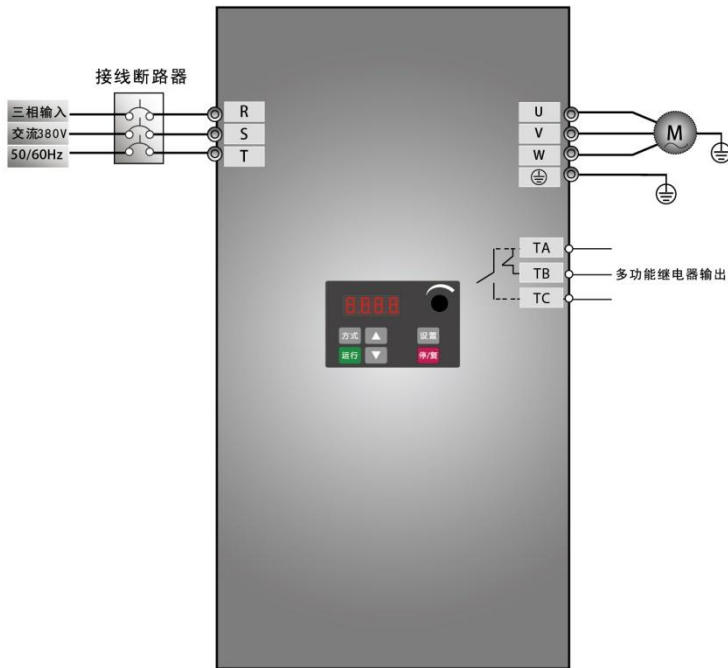
5-1 接线图 1
