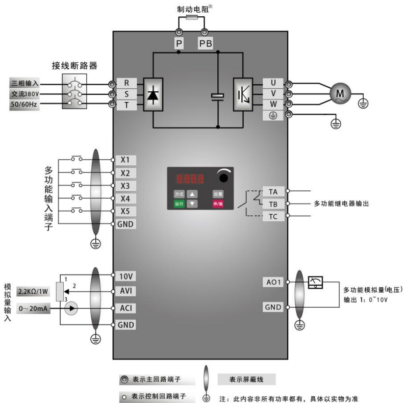
图 4-4 三相变频器标准配线图
