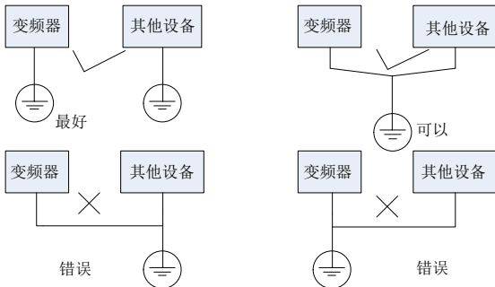
图 4-8 接地示意图
