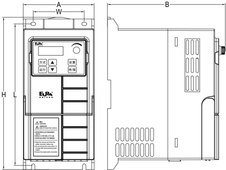
尺寸图
