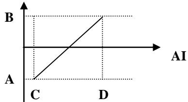
图 6-15 模拟给定与设定量的计算关系
