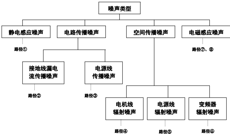
图 4-5 噪声类型图示
