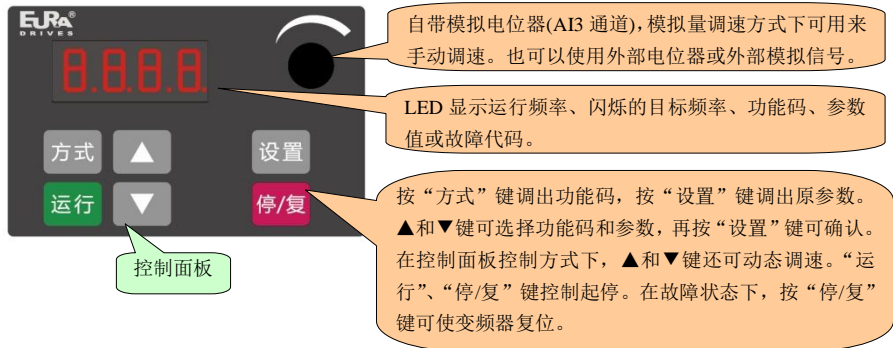
图 3-1 控制面板示意图
