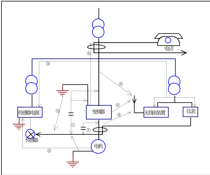
图 4-6 噪声传播途径
